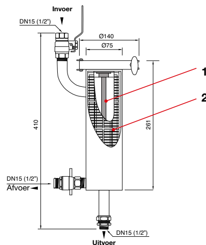
1. Magnetic rod
